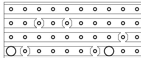
Côté circuit
